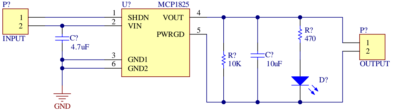
Şekil 1 Şematik Devre
